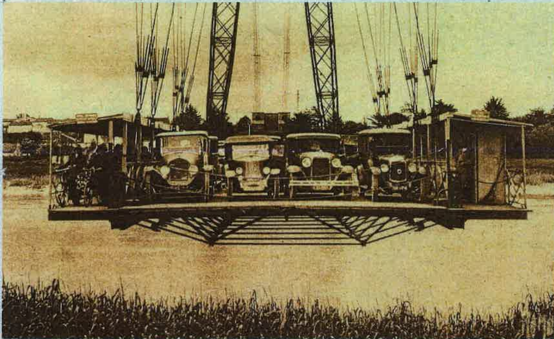
Puente de Rochefort entre las poblaciones francesas de Rochefort y Echillais. Foto: Puente Bizkaia
